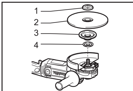
► 1. Contratuera 2. Disco flexible 3. Plato de goma 4. Brida interior
