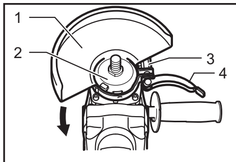
► 1. Carter de meule 2. Cage de roulement 3. Écrou 4. Levier
