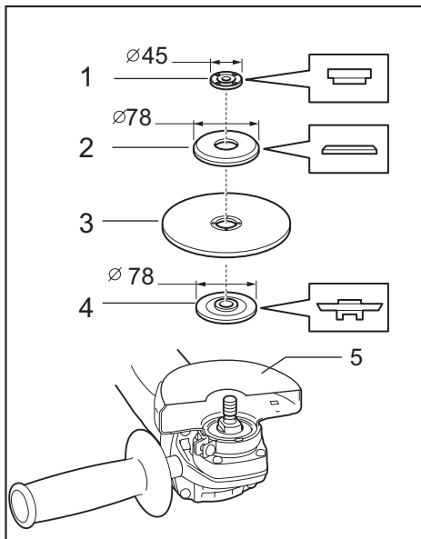
► 1. Contre-écrou 2. Flasque extérieure 78 3. Meule abrasive à tronçonner / roue diamantée 4. Bague interne 78 5. Carter de meule pour meule abrasive à tronçonner / roue diamantée
