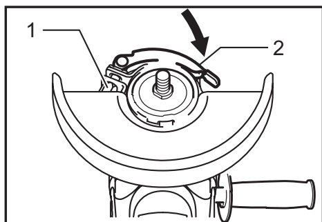
► 1. Nut 2. Lever
